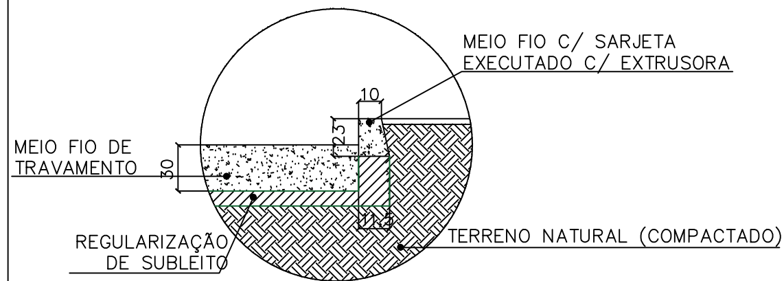
DETALHE 03 DETALHE MEIO FIO DE TRAVAMENTO
