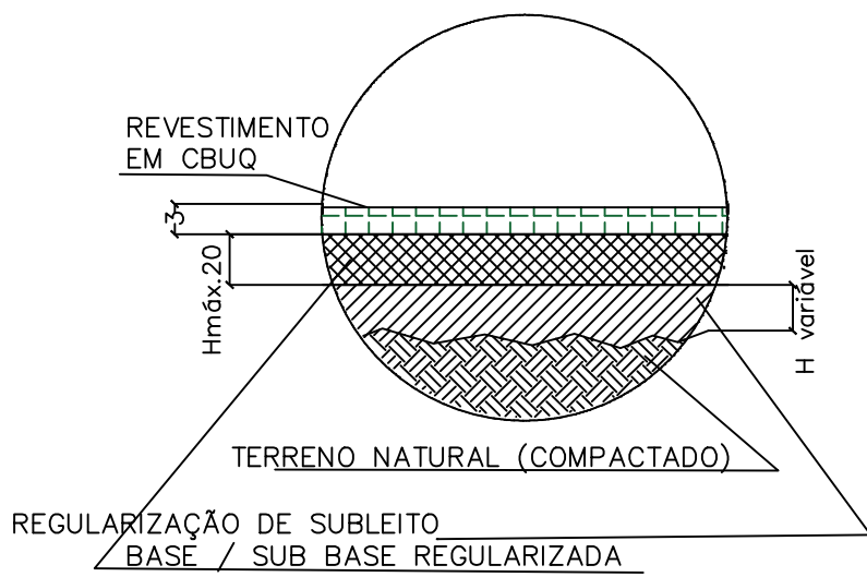
DETALHE 02 CAMADAS DA PAVIMENTAÇÃO
