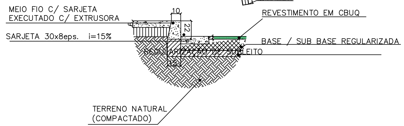
DETALHE 01 DETALHE DE SARJETA
