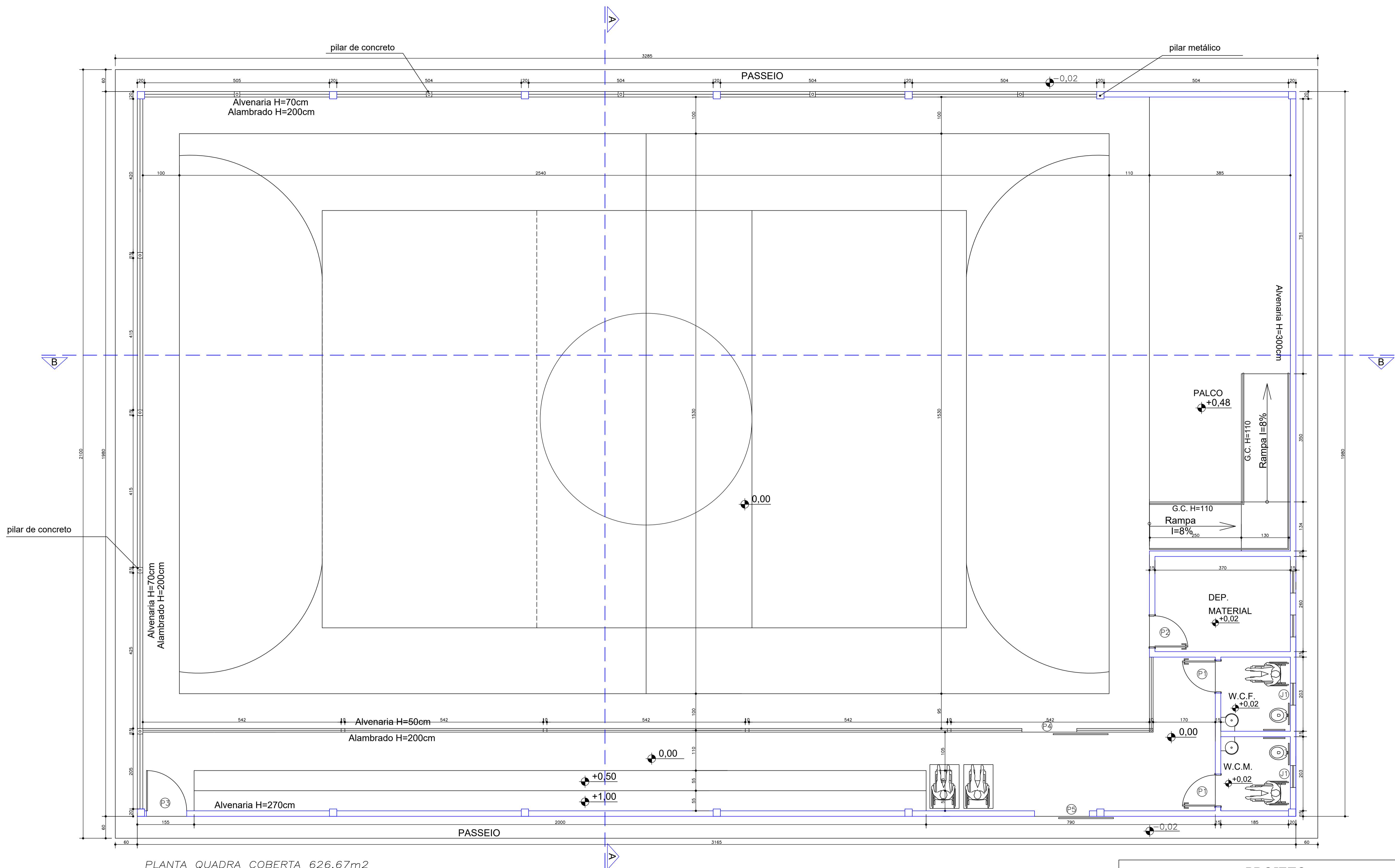
PLANTA QUADRA COBERTA 626,67m 2 ESCALA 1:50
