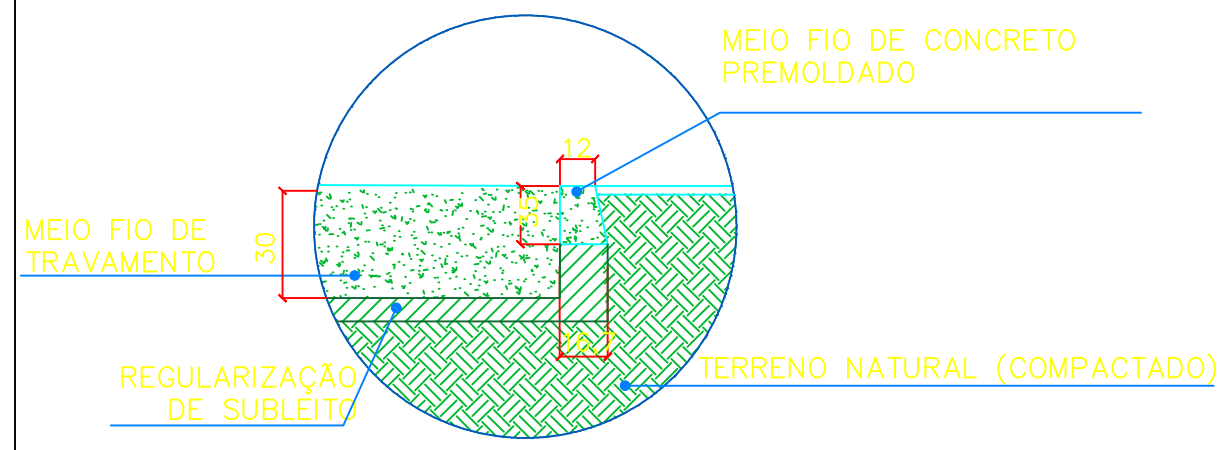
DETALHE 03 DETALHE MEIO FIO DE TRAVAMENTO
