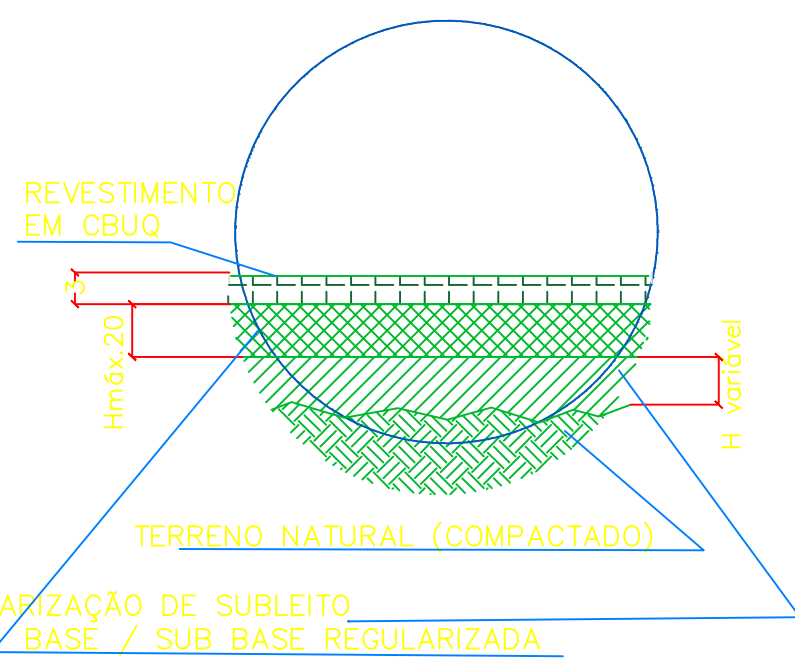
DETALHE 02 CAMADAS DA PAVIMENTAÇÃO
