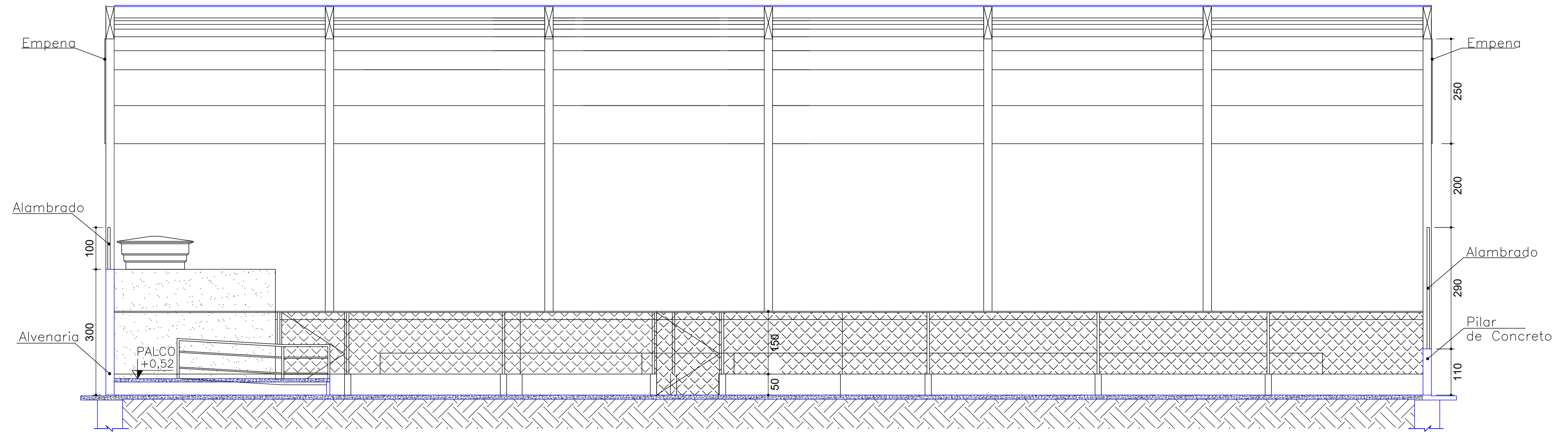
CORTE B-B Escala 1/100
